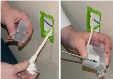
Installing Power Cable Instalar el Cable de alimentación
