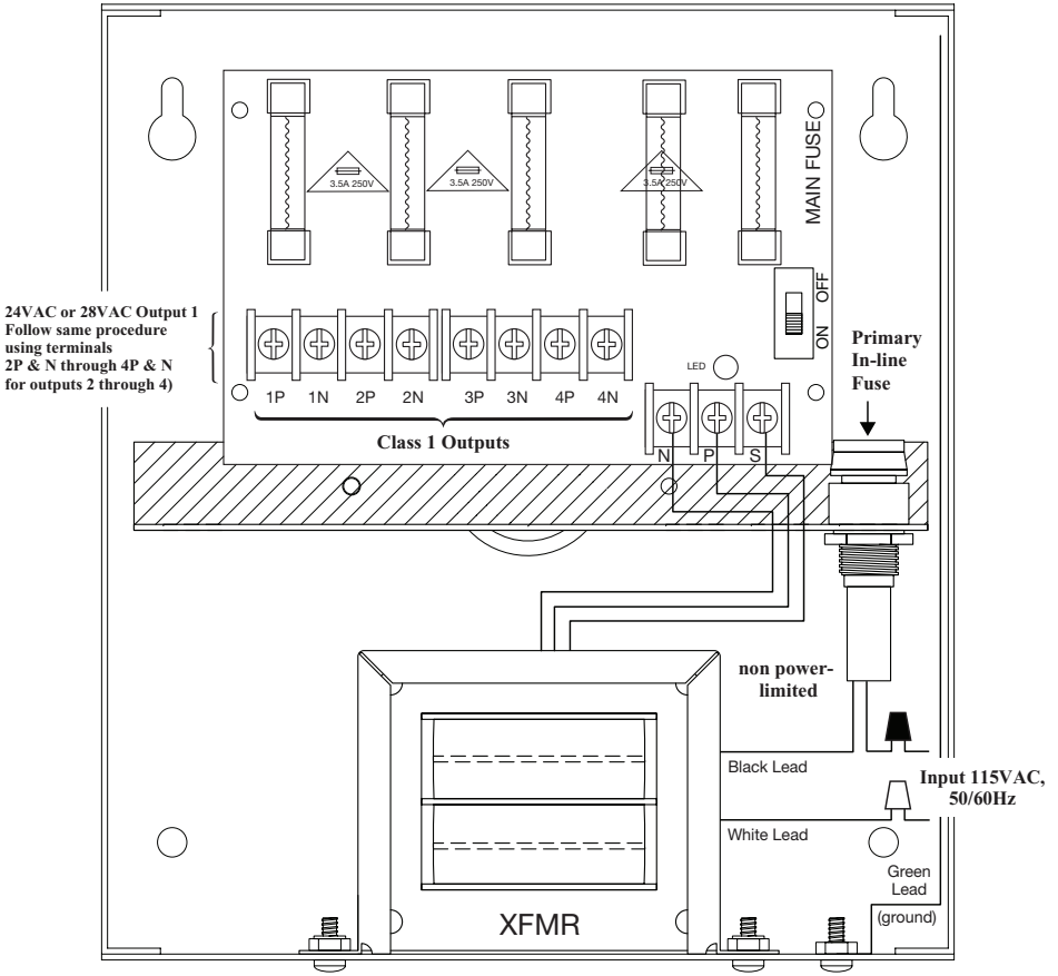
Fig. 1 - ALTV244UL
