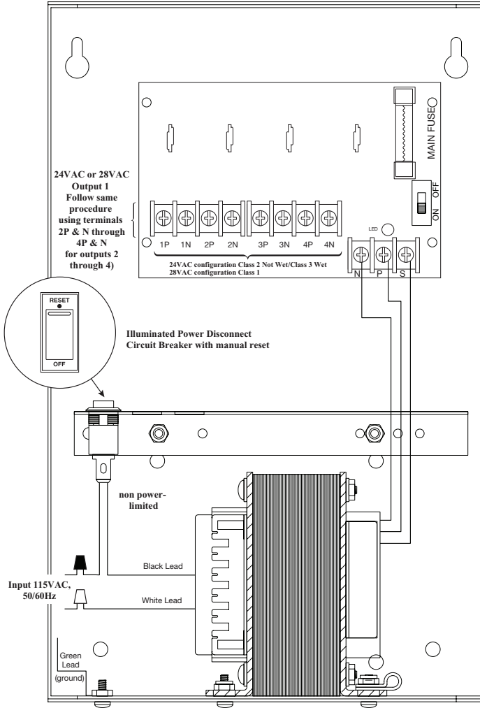
Fig. 5 - ALTV244175ULCB
