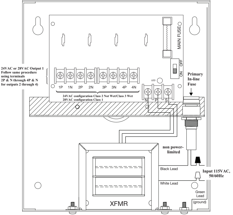
Fig. 2 - ALTV244ULCB
