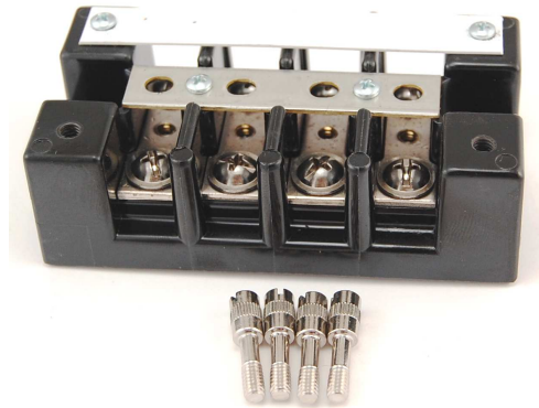
4 pole shown
